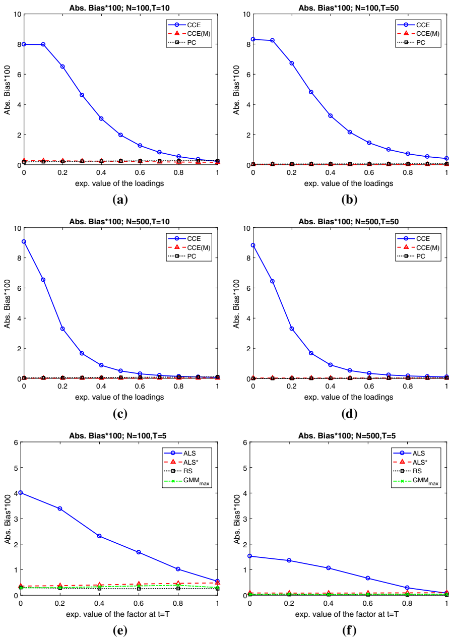
Fig. 1 Normalization failure for CCE (DGP1) and ALS (DGP2)
