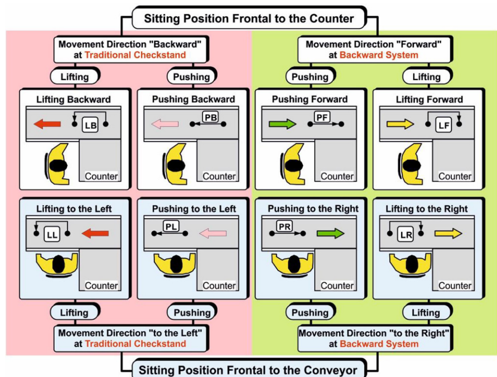
Fig. 29 Sitting position frontal to the counter ( upper half ) or frontal to the conveyor ( lower half ) in conventional check-stands with backward movements of the left hand-arm-system or movements “to the left” ( upper and lower left part ) and in ergonomically designed check-stands with movements “to the right” ( lower right part ) Abb. 29 Sitzposition frontal zur Kassenbox ( obere Hälfte ) oder frontal zum Förderband ( untere Hälfte ) bei konventionellen Kassenständen mit Bewegungen des linken Hand-Arm-Systems „nach hinten“ bzw. „nach links“ ( oben und unten links ) und bei ergonomisch neu gestalteten Kassen-Arbeitsplätzen mit Bewegungen (des linken Arms) „nach rechts“ ( unten rechts )
