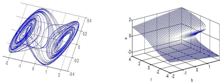
a. chaos
