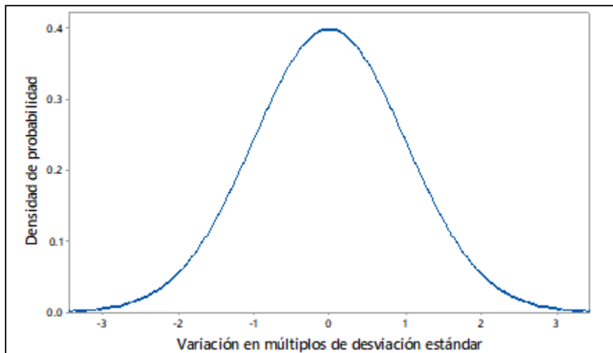
Gráfica 4. Representación de una distribución normal.
