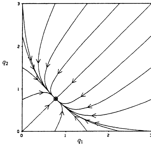
Abbildung 2: Flußlinien der Qualitätsvariablen q_j für \gamma \ll 1 und für Wettbewerbsfähigkeit \phi = 0,8\phi_C . Die Flußlinien nähern sich einem einzigen stationären Zustand.
