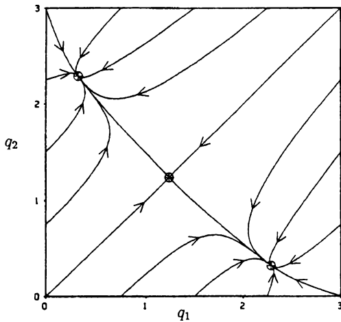
Abbildung 3: Flußlinien der Qualitätsvariablen q_j für \gamma \ll 1 und für Wettbewerbsfähigkeit \phi = 1,2\phi_C . In Abhängigkeit vom Anfangszustand nähern sich die Flußlinien einem von zwei stabilen stationären Zuständen.
