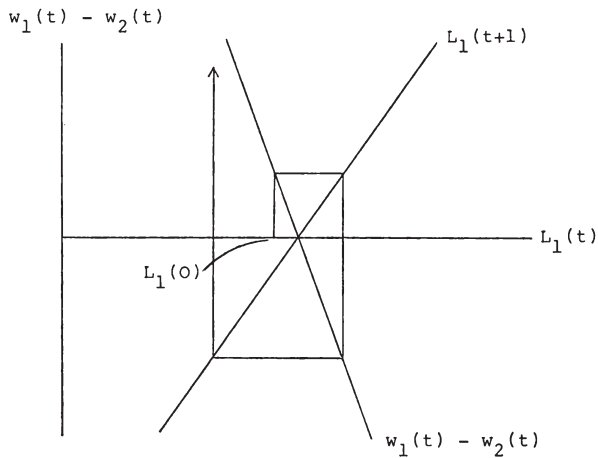
Abb. 4. Instabiler Wanderungsprozeß.
