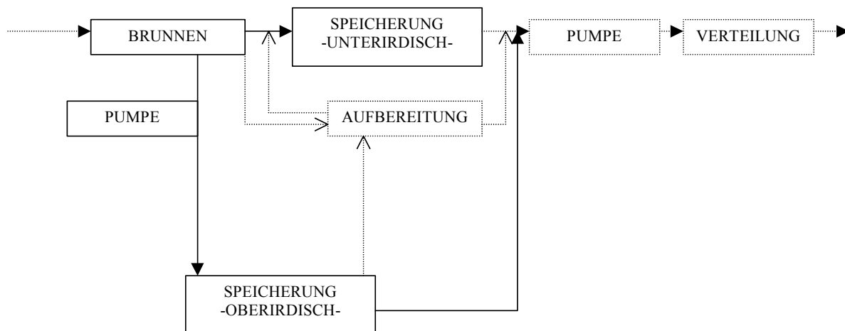
Abbildung 4: Wasserspeicherung
