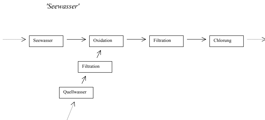
Abbildung 3b: Aufbereitung von Seewasser
