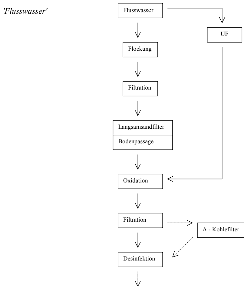
Abbildung 3a: Aufbereitung von Flusswasser
