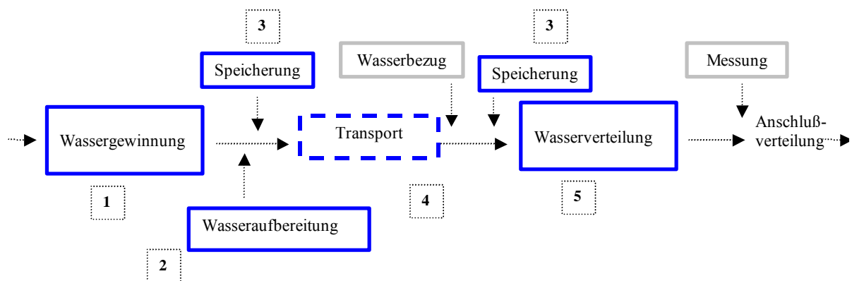
Abbildung 1: Die Produktionsstruktur eines Wasserversorgers
