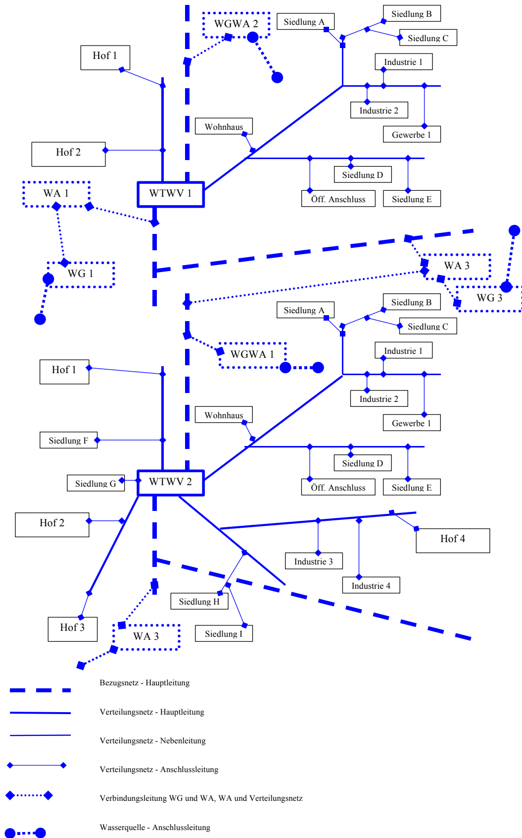
Abbildung 20: Skizze eines ländlichen 'Pool-Modells'
