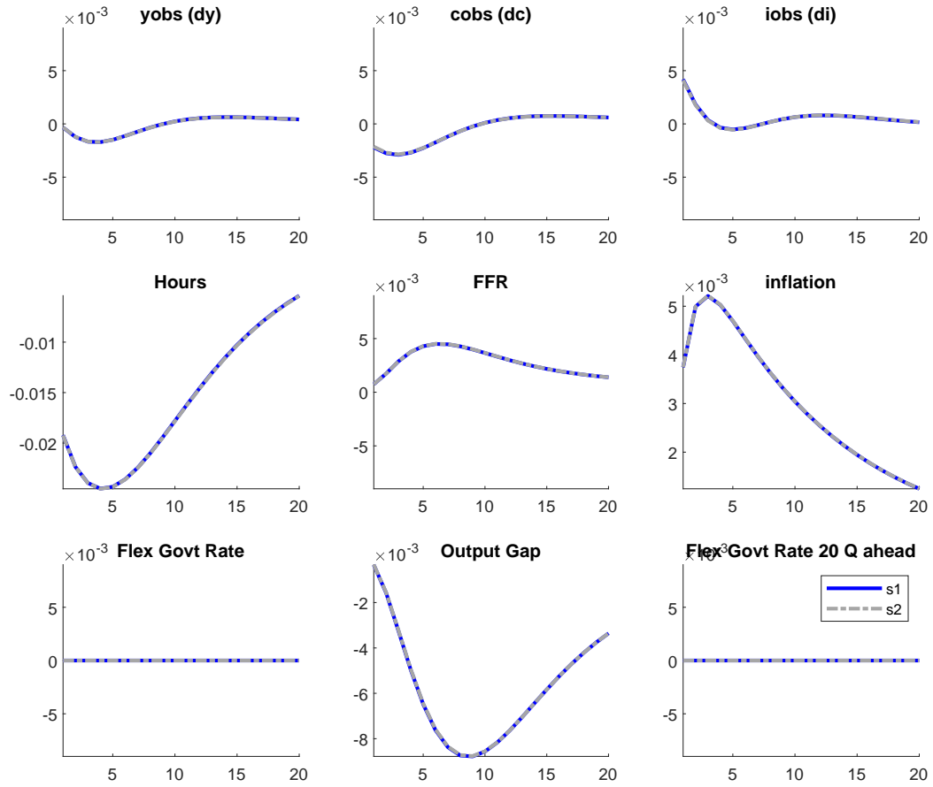
Figure 8: WageMarkup
