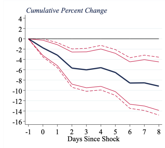
(d) Algorithmic
