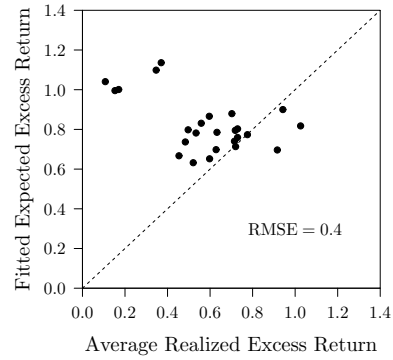
(d) FF3 Model + MOM + NMP
