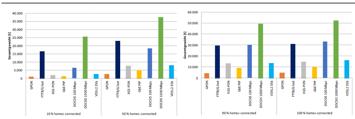
Abbildung 4-16: Gesamtgewicht der jeweiligen Zugangstechnologien (in t)
