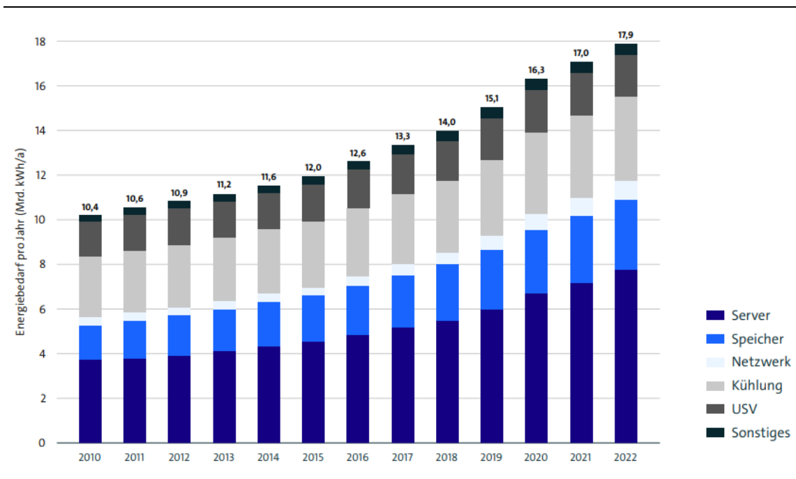
Abbildung 4-4: Energiebedarf der Rechenzentren in Deutschland
