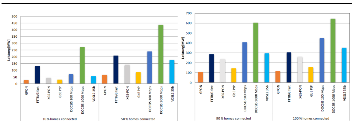
Abbildung 4-15: Leistungsaufnahme der jeweiligen Zugangstechnologien für eine Gesamtversorgung Deutschlands (in MW)
