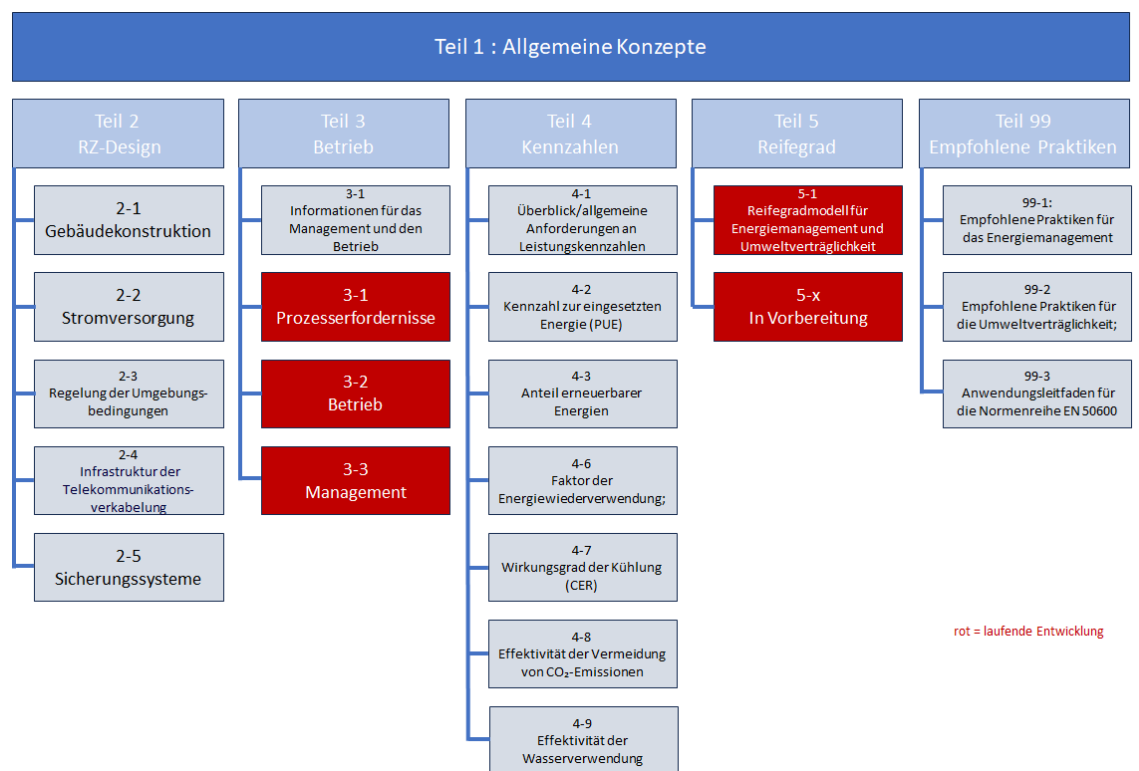
Abbildung 4-6: Ausgestaltung der EN 50600
