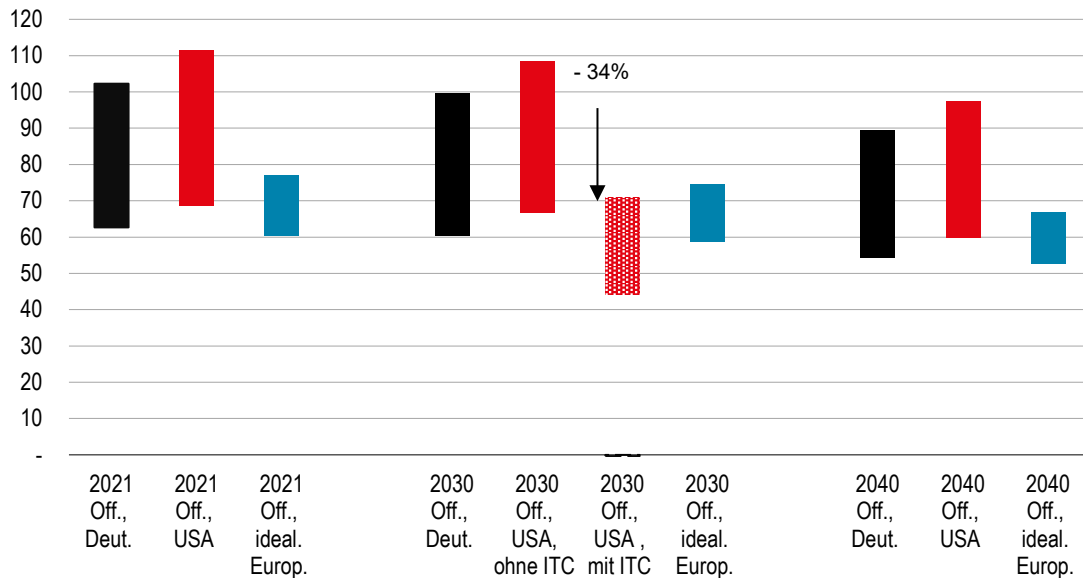
Abbildung 3: Projektion der Stromgestehungskosten für Windkraftanlagen Offshore in Euro 2021 /MWh
