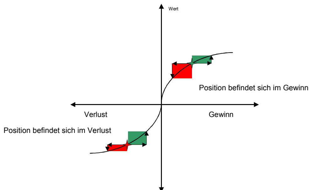
Abbildung 2: Wertefunktion der Prospect Theory
