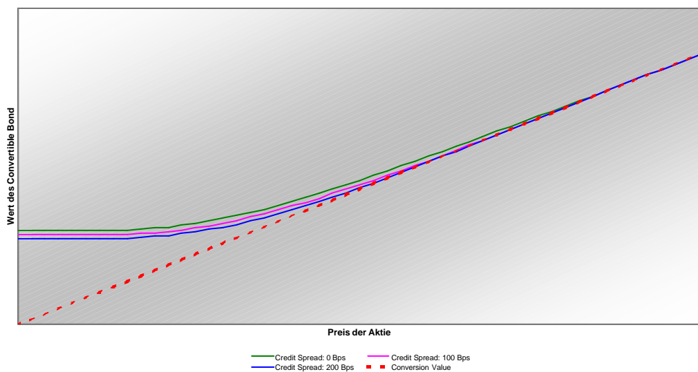
Abb. 5 Wertverlauf eines Convertible Bonds bei verschiedenen Credit Spreads
