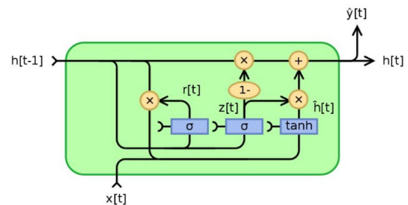
Fig. 2 GRU architecture
