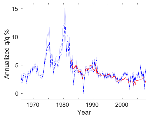
(d) AR(2)
