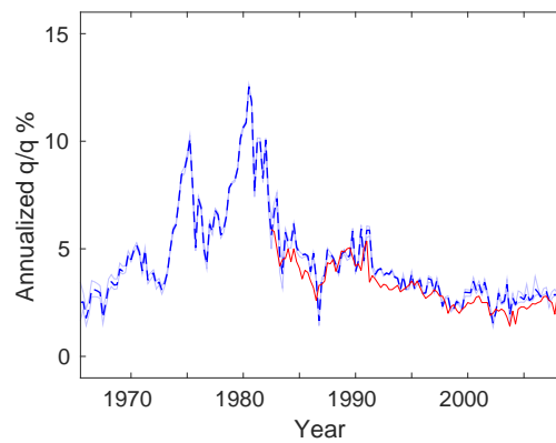
(b) SAC
