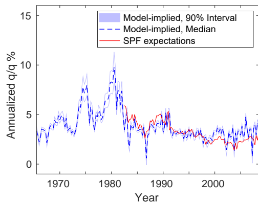
(a) BLE
