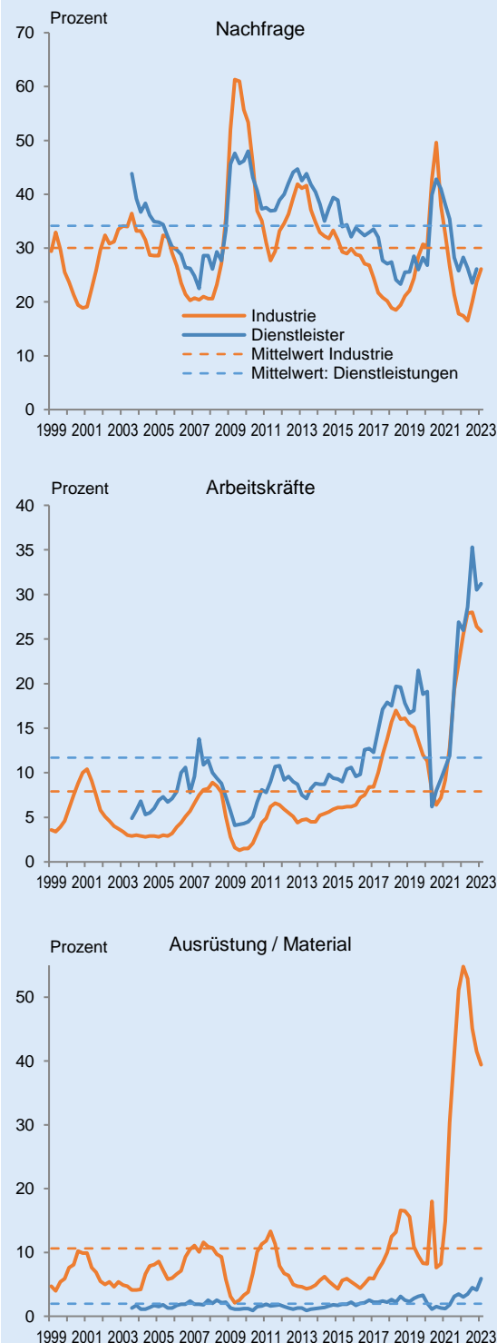
Abbildung 8: Produktionslimitierende Faktoren
