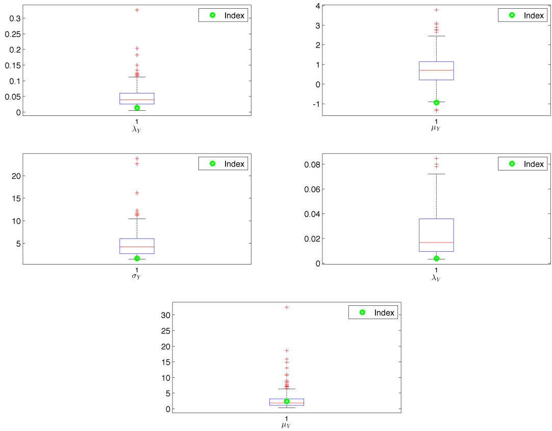
Figure 1: Parameter Box Plots (SVIJ Model)
