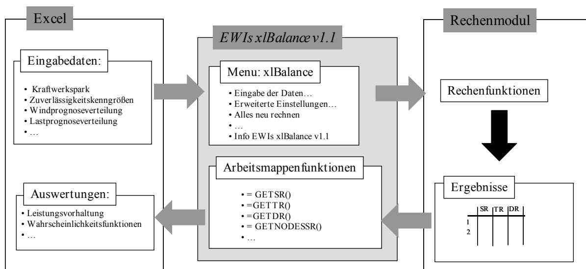
Abbildung 12: Benutzung und Funktionsweise von xlBalance
