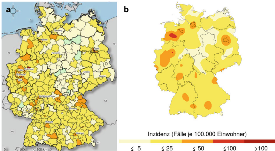
Abb. 7 Darstellung der Corona-Infektionslage am 3. Oktober 2020 ( Quelle : Tagesbericht des RKI (a) und alternative Darstellung (b) über Kerndichteschätzer). Benutzung der RKI-Farbskala
