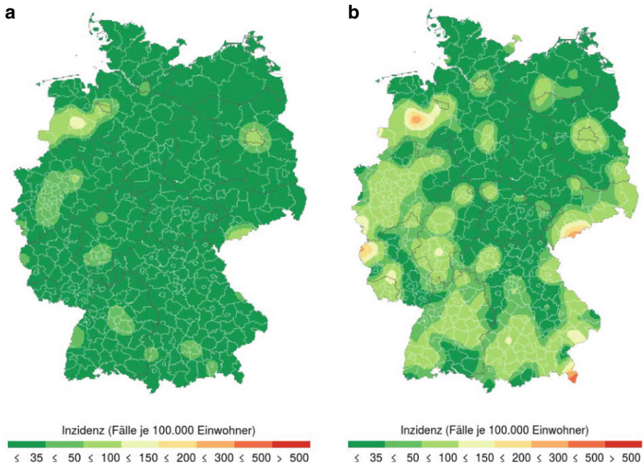
Abb. 1 Geschätzte lokale 7-Tages Inzidenz am Beginn der 2. Pandemie-Welle in Deutschland. a Periode 02.10.2020–08.10.2020 b Periode 13.10.2020–19.10.2020. (Darstellung https://www.inwt-statistics.de/blog-artikel-lesen/COVID-19_Karte_der_lokalen_7-Tage-Inzidenz_im_Zeitverlauf.html )
