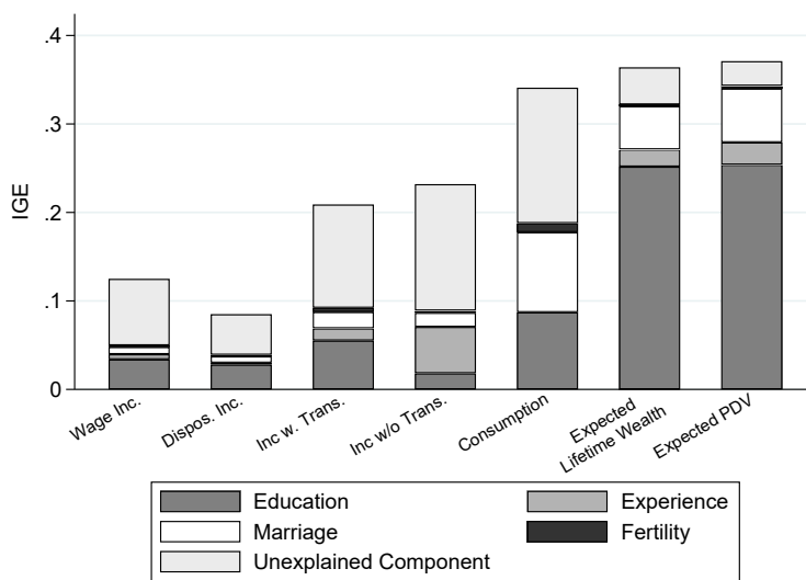
(b) IGE Decomposition
