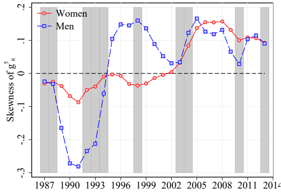
(a) Kelley Skewness
