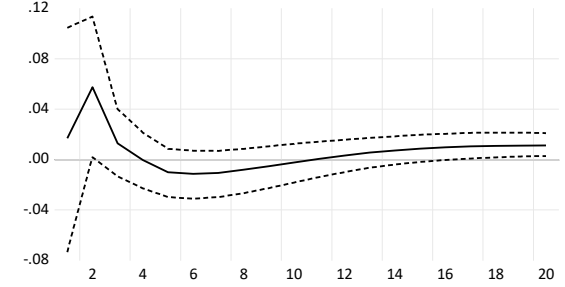
(d) Response of \Delta\pi_t to an i_t shock, 2004Q4
