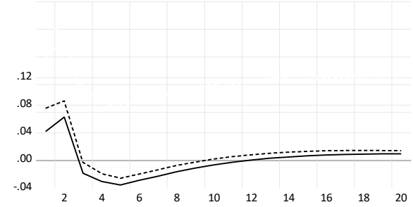
(d) Response of \Delta\pi_t to an i_t shock, craft production system
