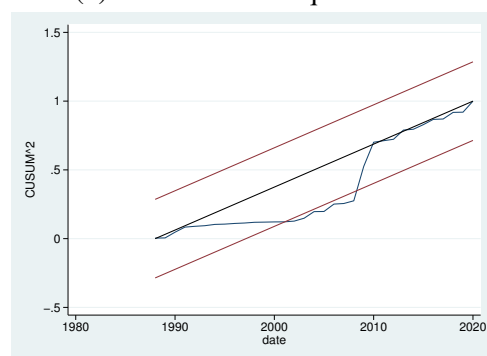
(d) Silver CUSUM squared test
