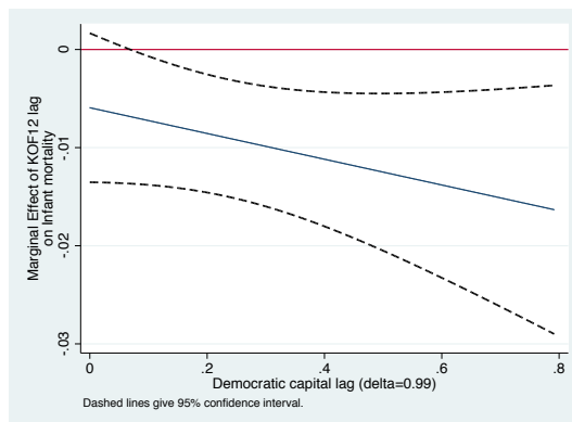
(d) Democratic capital ( \delta = 0.99 )
