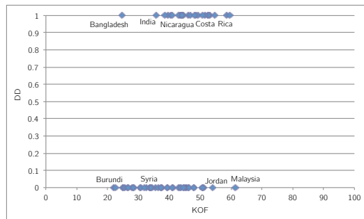
(b) KOF and DD
