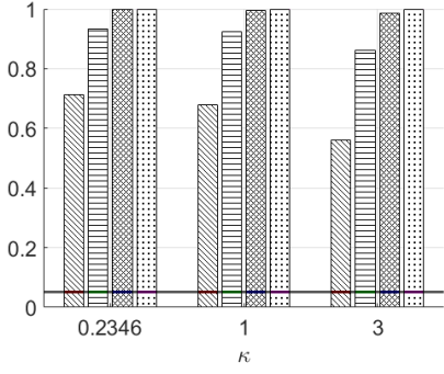
(d) \mathbb{H}_0 : \beta(1) = \beta(2) , \rho = 0.5, p = 1
