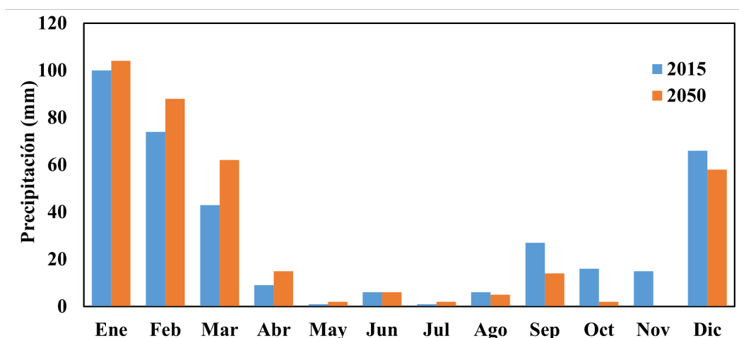
Figura 6: Precipitación acumulada 2015 y 2050 - Patacamaya
