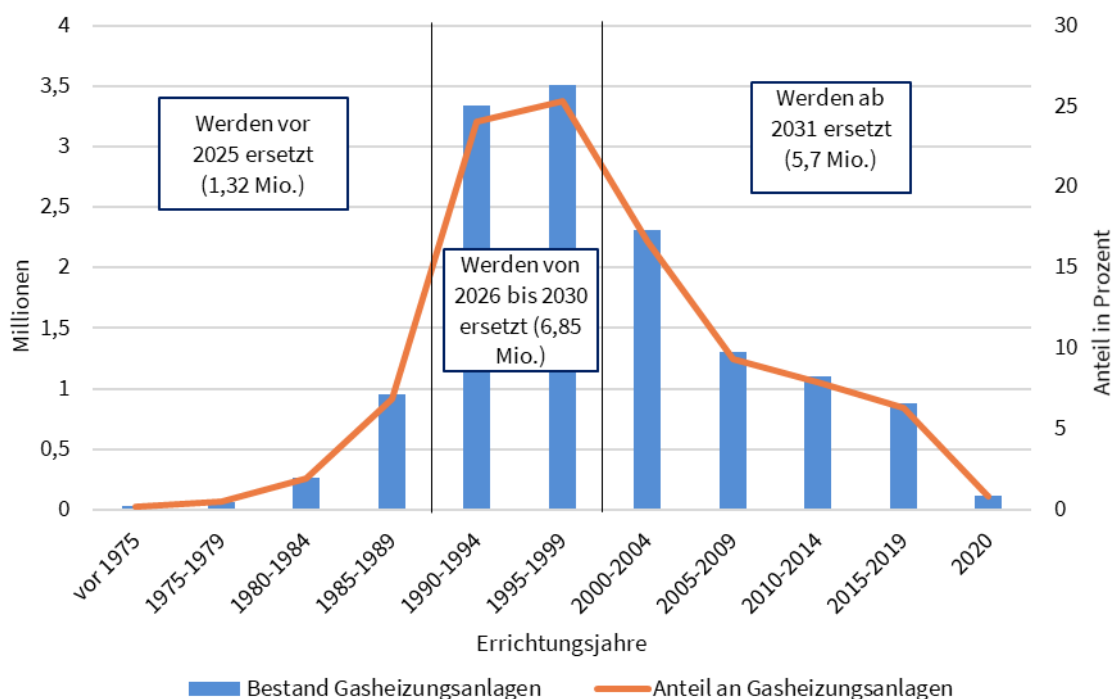
Abbildung 6: Bestand an Gasheizungen nach Errichtungsjahren und angenommene Ersetzungszeiträume
