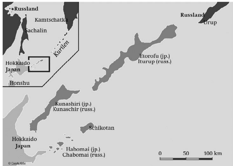
Karte 2 Umstrittene Inseln der Kurilen-Kette
