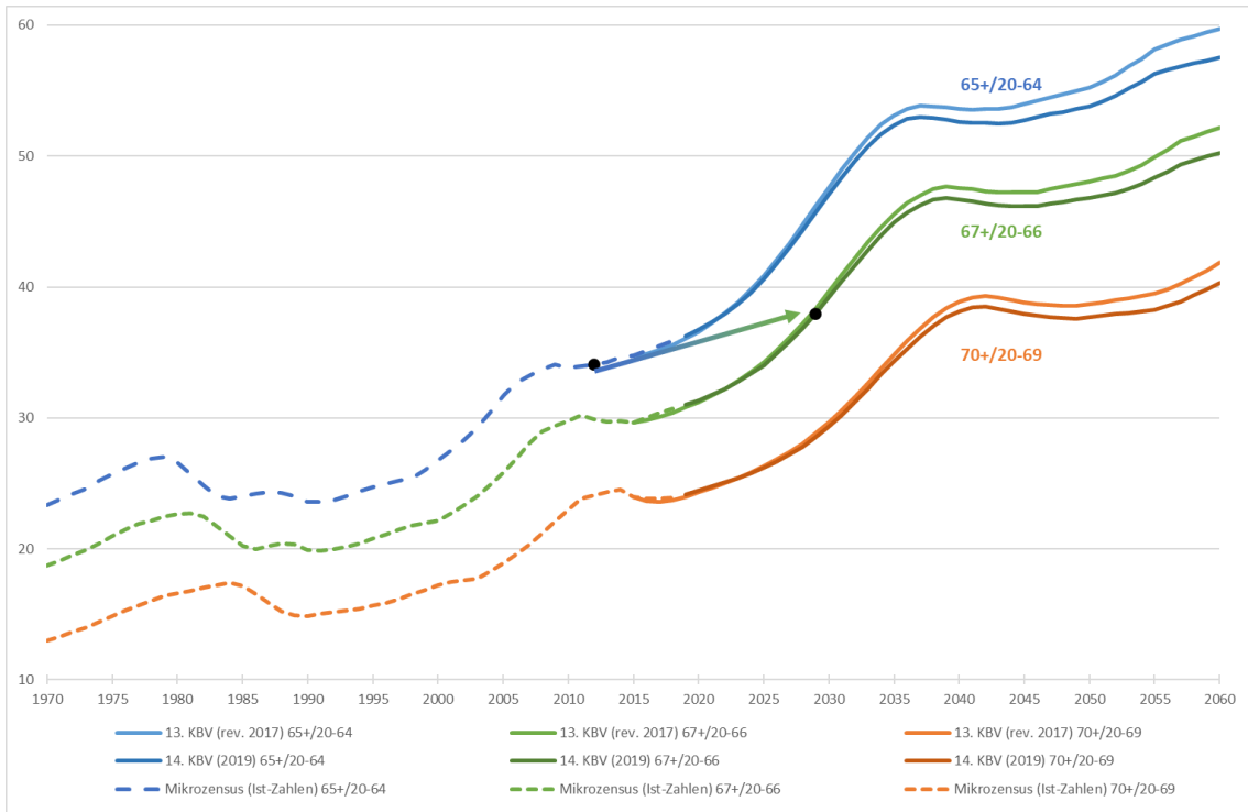
Abbildung 2: Altenquotienten (Deutschland, 1970-2060)
