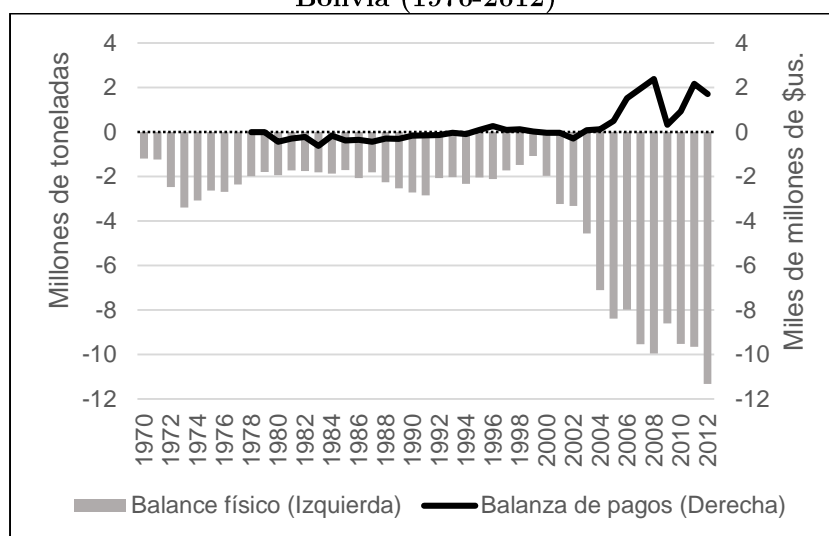
Gráfico 2: El balance comercial físico y el saldo global de la balanza de pagos para Bolivia (1970-2012)
