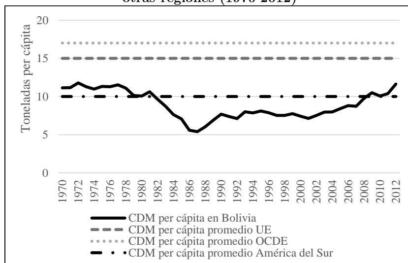
Gráfico 4: Consumo doméstico de materiales per cápita para Bolivia con respecto a otras regiones (1970-2012)
