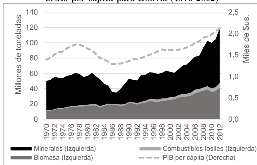
Gráfico 1: El consumo doméstico de material por categorías y el producto interno bruto per cápita para Bolivia (1970-2012)
