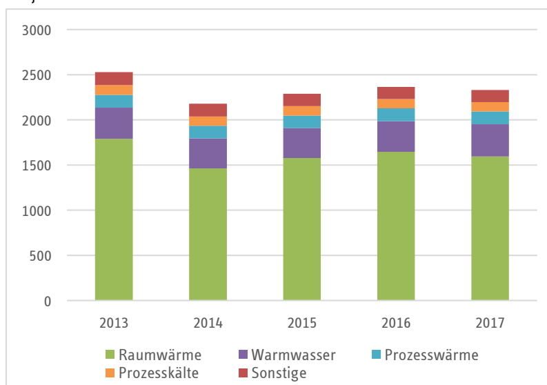
Abbildung 4: Energieverbrauch nach verschiedenen Anwendungen im Haushaltssektor in PJ
