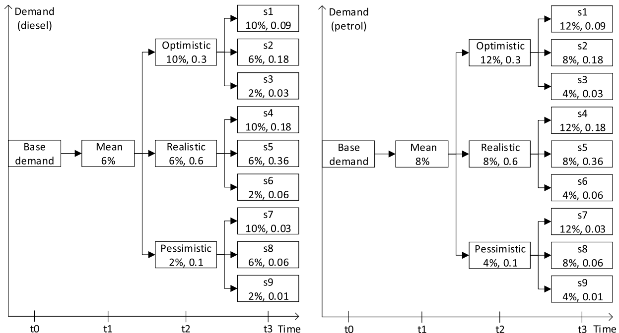
Fig. 4. Scenario trees.
