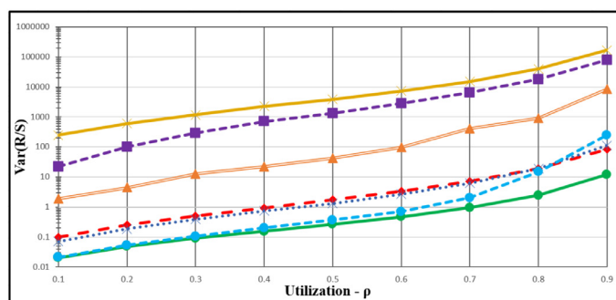
(d) \text{Var}(R/S) vs Utilization
