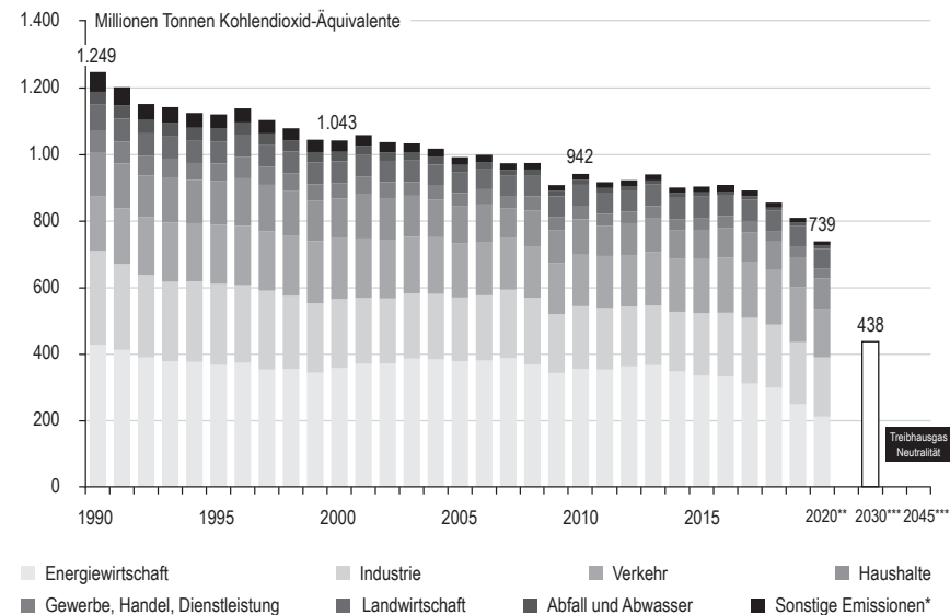
Abbildung 5: Emissionen der von der UN-Klimarahmenkonvention abgedeckten Treibhausgase
