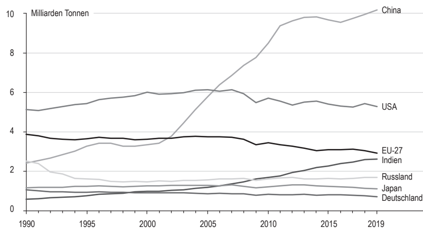
Abbildung 6: Jährliche CO 2 -Emissionen aus der Verbrennung fossiler Brennstoffe für die Energie- und Zementproduktion*
