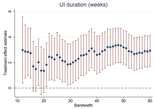
(d) 2 nd -order polynomial
