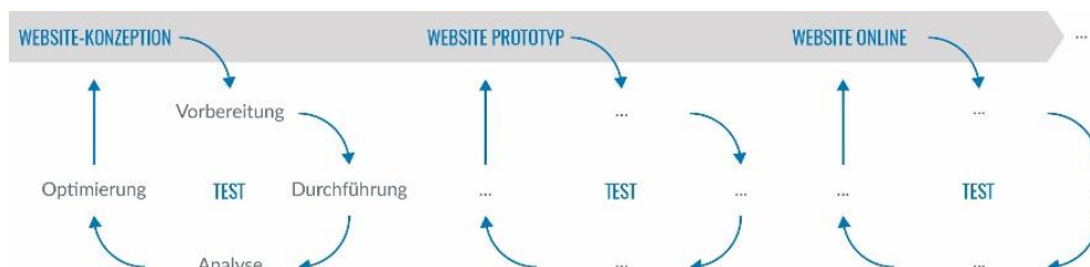
Abbildung 1: Iteratives Testen 82
