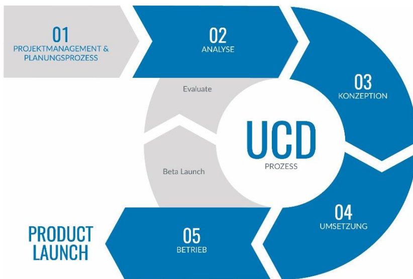
Abbildung 13: UCD-Prozess 95
