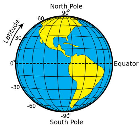
Fig. 3. Latitude (geolounge, 2014).
