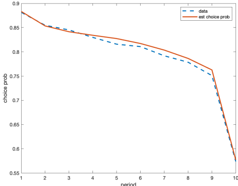
(b) DGP 2
