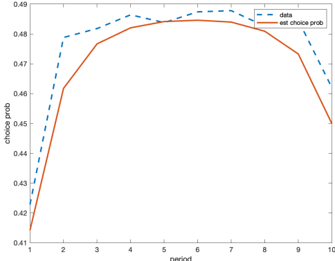
(d) DGP 4
