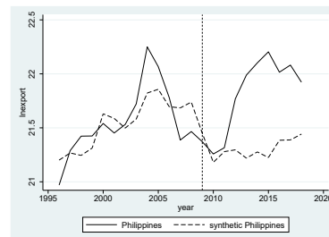
V (RMSPE 0.2041212)
