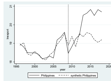
V (RMSPE 0.1524746)
