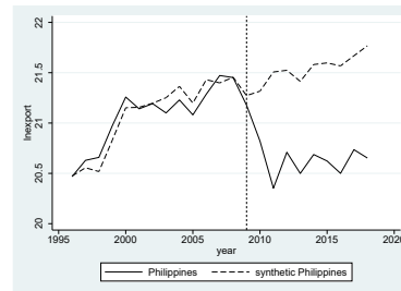
V (RMSPE 0.1030114)
