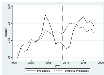
I. (RMSPE: 0.2276206)
