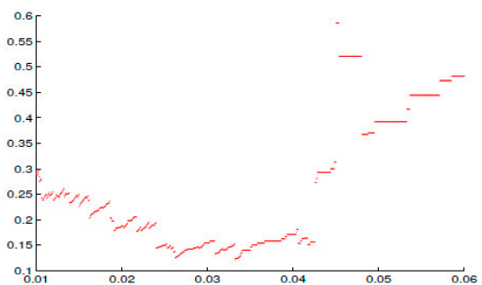
(d) MICEX external index.
