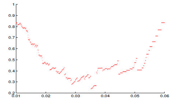
(d) TASI extremal index.
