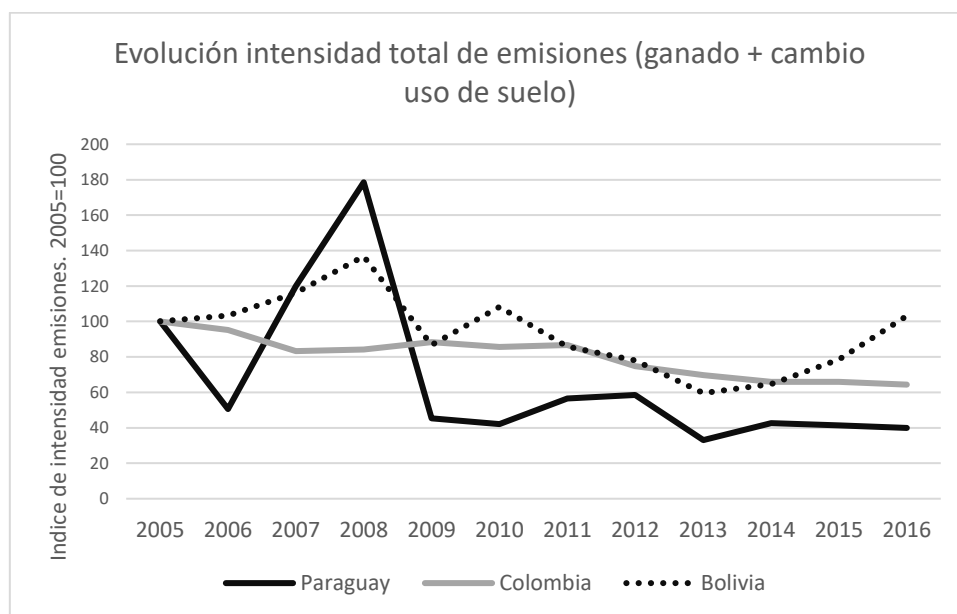
Gráfico 5. Evolución de la intensidad de emisiones totales. Originadas en el stock ganadero y por efecto de cambio en el uso del suelo
