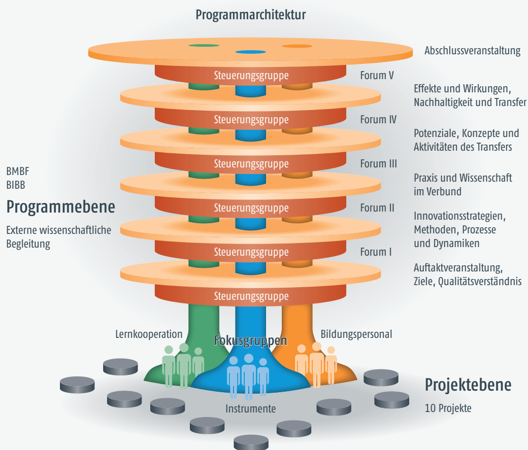
Abbildung 4 Programmarchitektur
