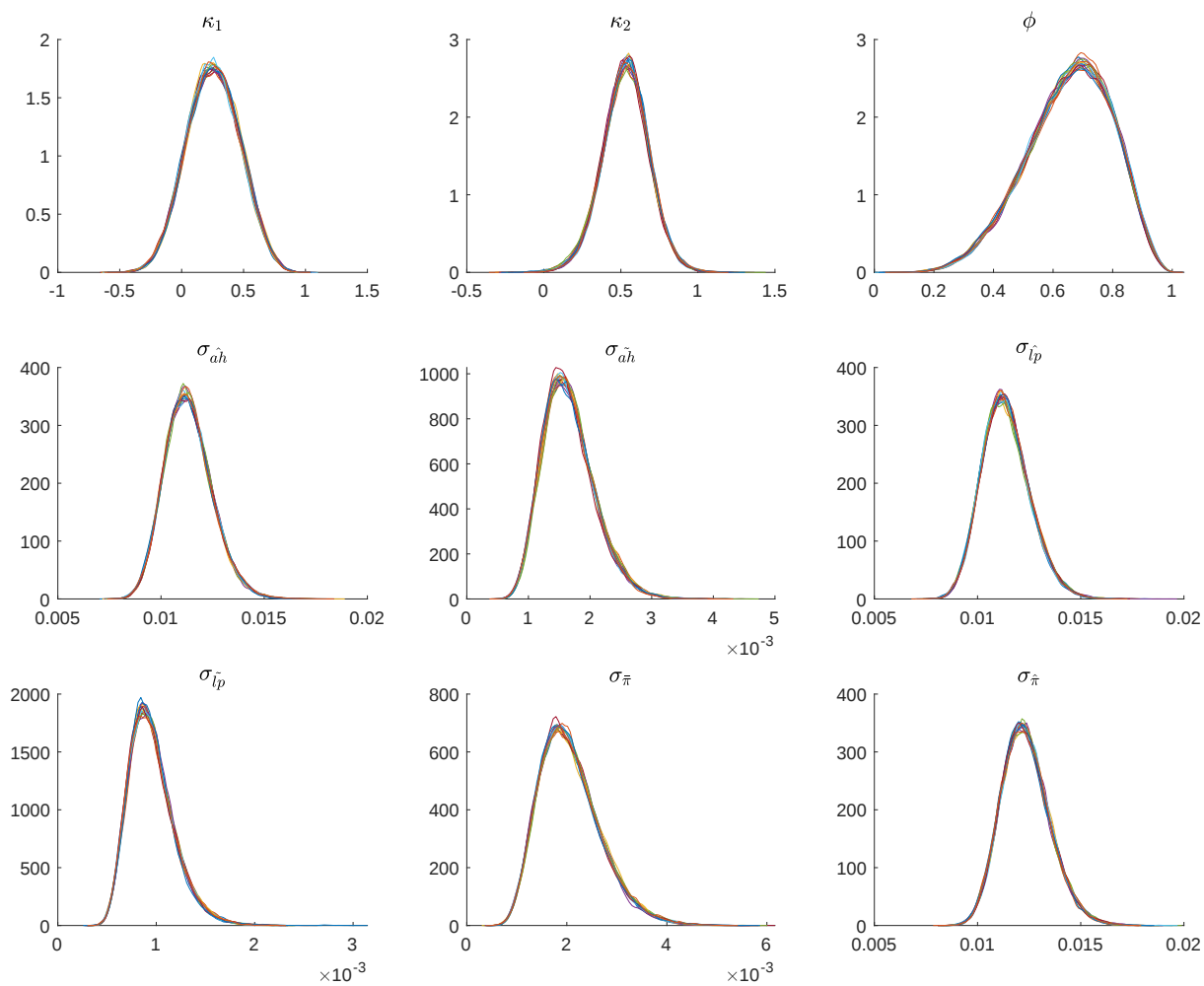
Figure B5: Posterior distributions - parallel posterior chains (model A)
