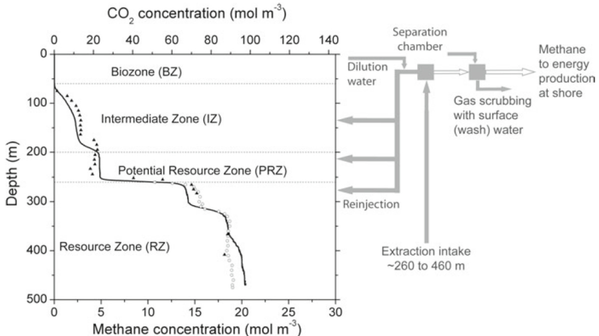
Abb. 9: Angenommene Methankonzentration in den jeweiligen Zoen und Modell des Extraktionsvorgangs von Methan und Reinjektion des Tiefenwassers (WUEST et al. 2012)
