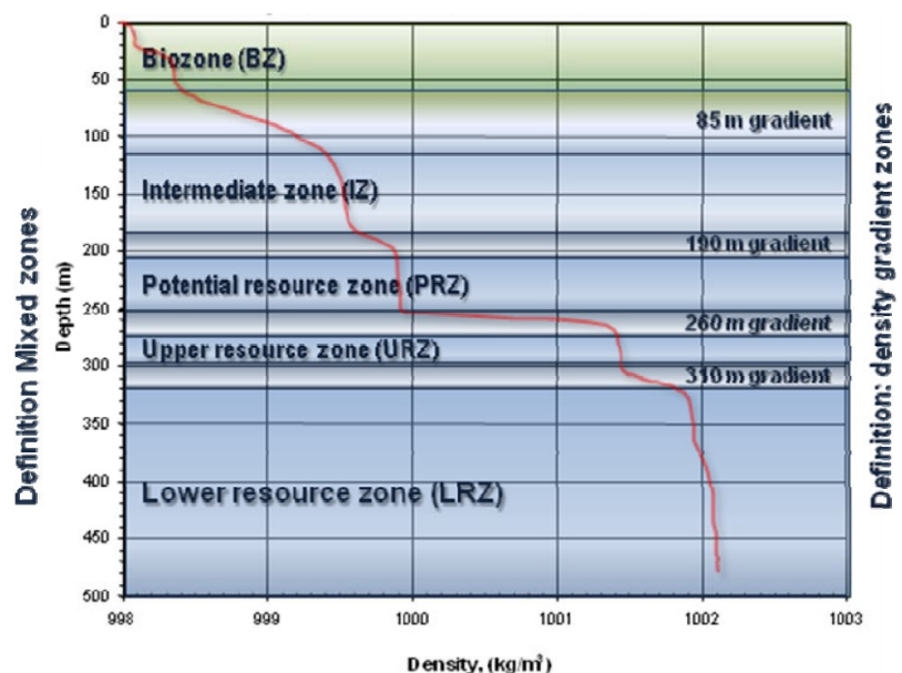
Abb. 3: Vertikales Sättigungsprofil, mit den jeweiligen Zonen des Lake Kivu (EWGLKGE 2010, S. 6)
