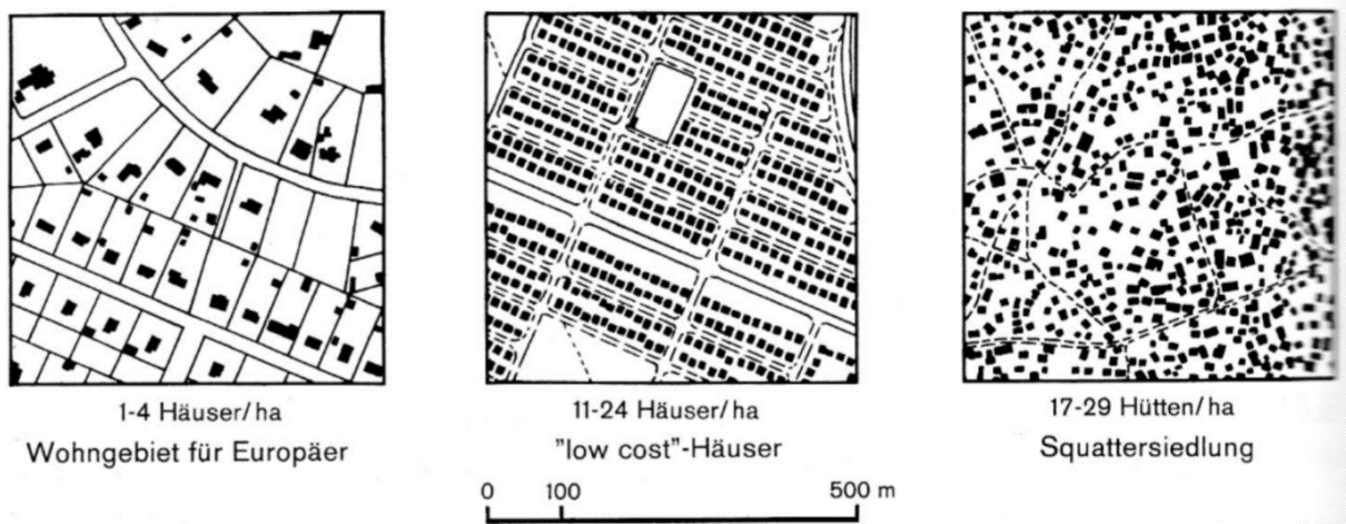
Abb. 5: Typische Bebauungsstrukturen in Subsahara-Afrika (WILLIAMS 1984)
