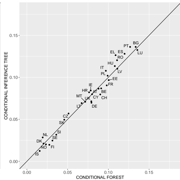
(d) Conditional Inference Tree
