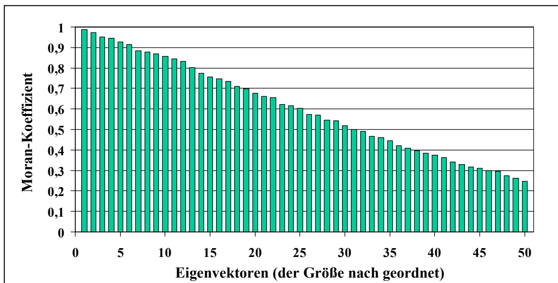
Abb. 1: Substantielle Moran-Koeffizienten
