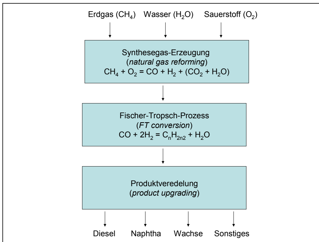
Abbildung 5: Fischer-Tropsch-Prozess 24
