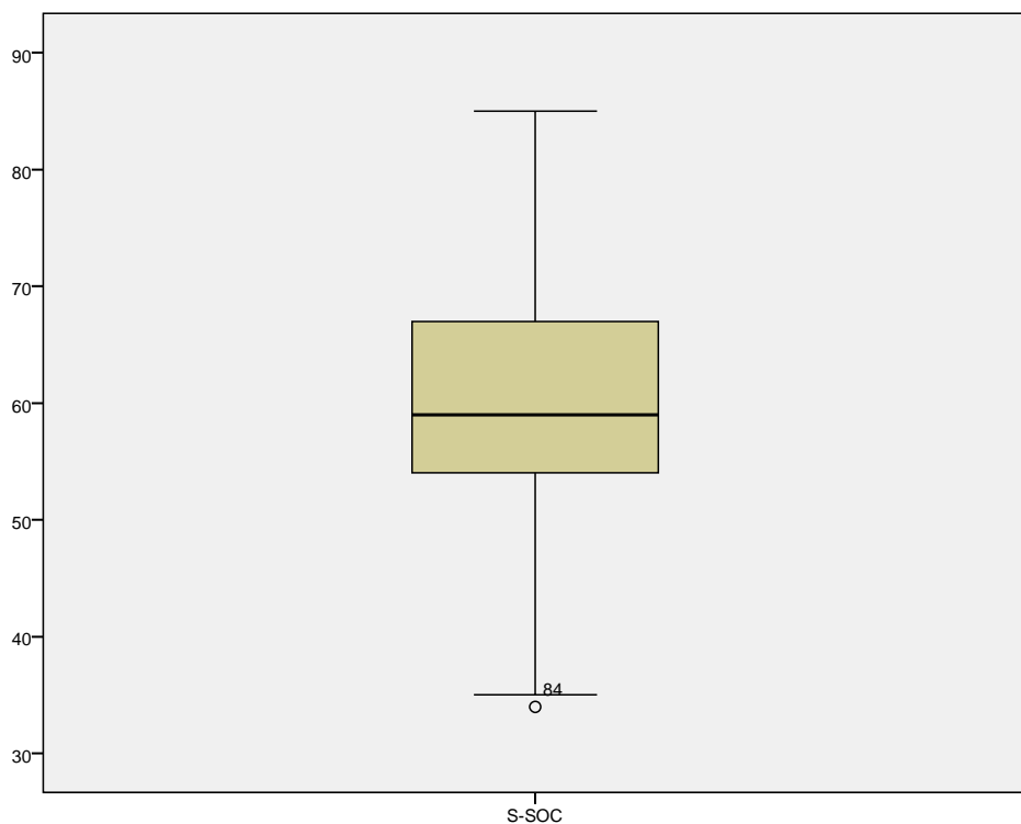
Abbildung 4: Boxplot S-SOC
