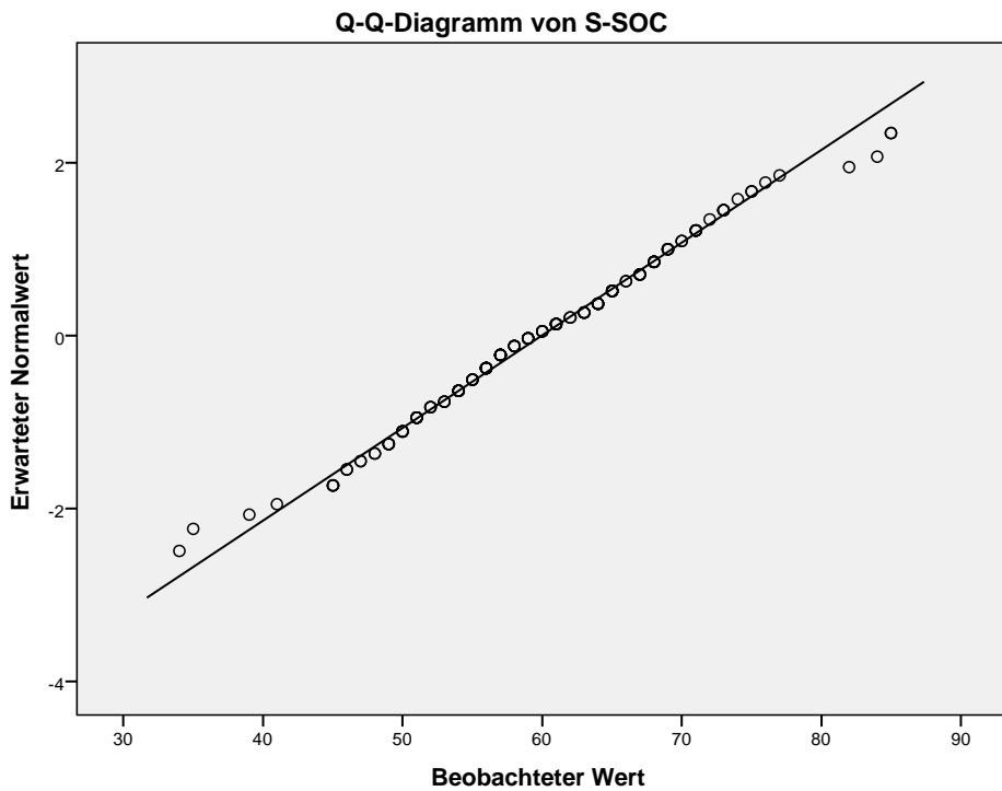
Abbildung 3: Q-Q-Diagramm S-SOC
