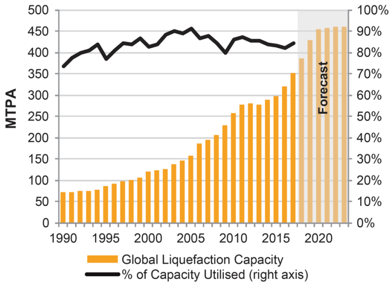
Figure 10: Global existing LNG liquefaction capacity and utilisation
